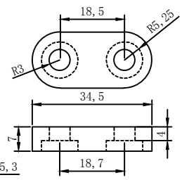
陶瓷垫片一
