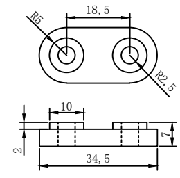
陶瓷垫片二
