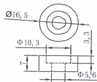
圆陶瓷垫片
